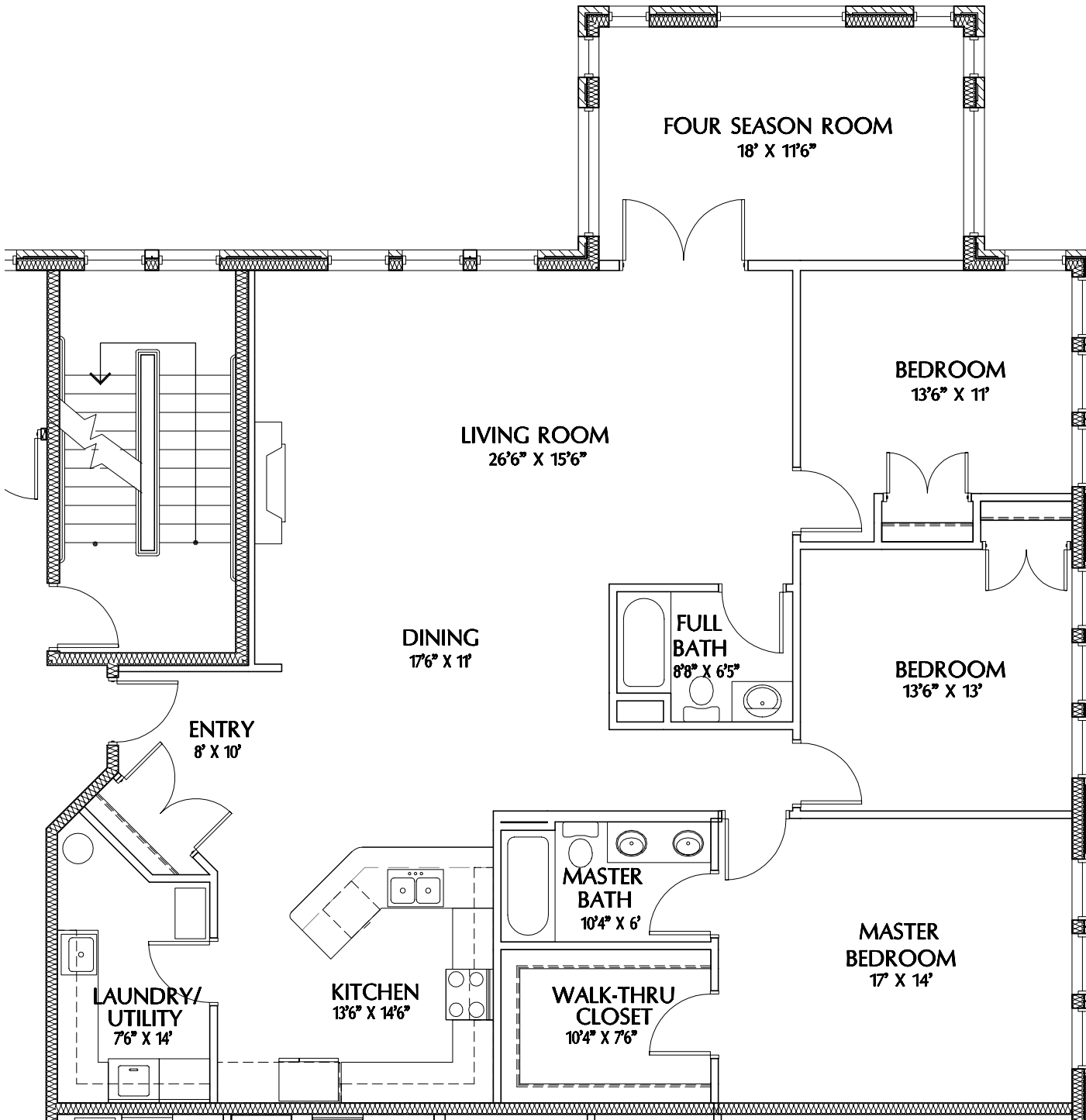
3 BEDROOM - 2 BATH - OAK 2,059 S.F.
